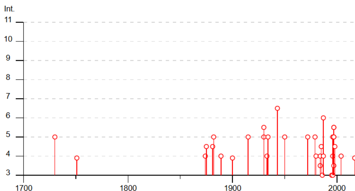
Fig. 12: schema sismo storico del comune di Ripatransone
