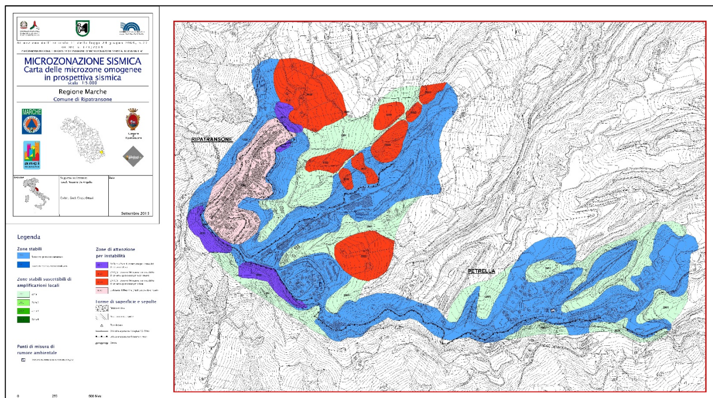
Fig. 15: stralcio carta delle MOPS – MS livello III comune di Ripatransone
